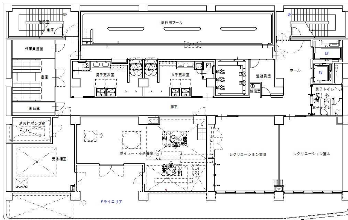
B1階 平面図
