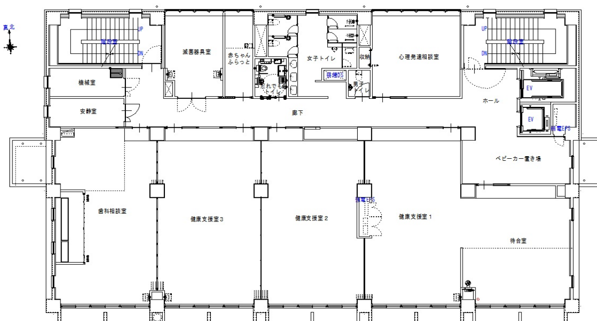
2階 平面図
