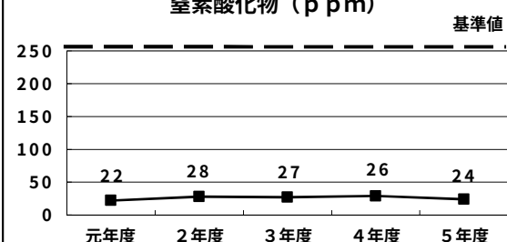
3号炉 窒素酸化物 (ppm)
