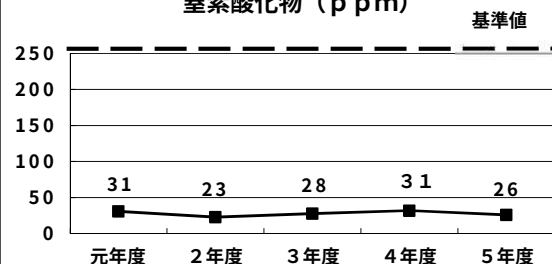
2号炉 窒素酸化物 (ppm)
