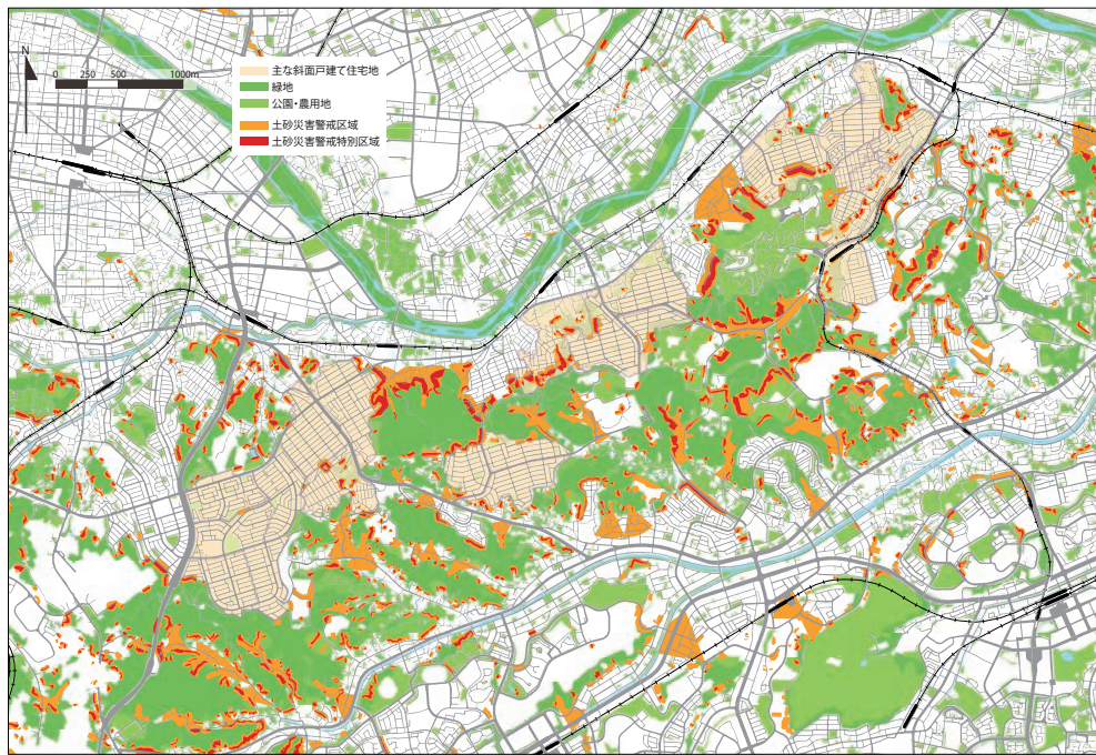
多摩の長山に開発された丘陵斜面住宅地と土砂災害警戒区域
