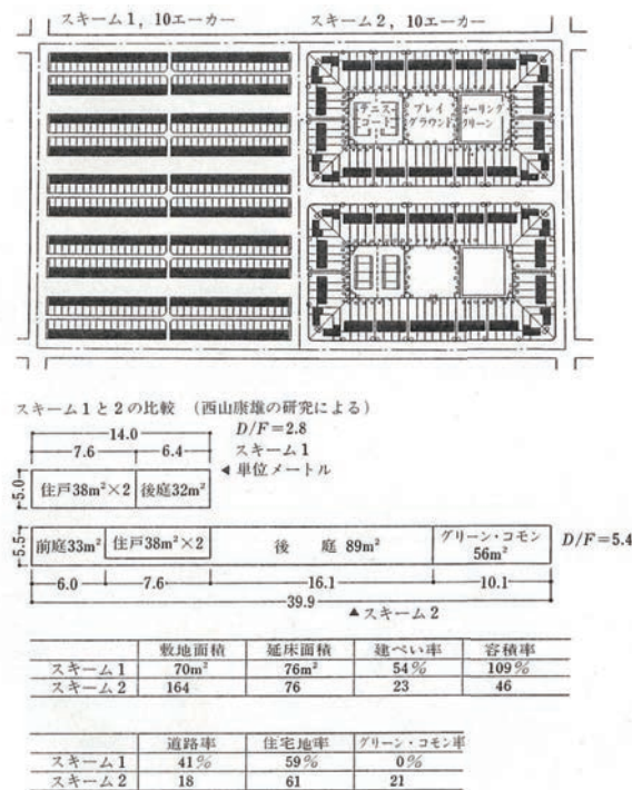
図5.8 建築条例住宅の一例(スキーム1)とアンウィンの改善案(スキーム2)
