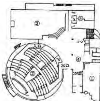
1階平面図
