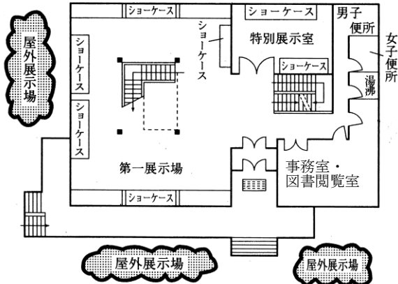
1階平面図
