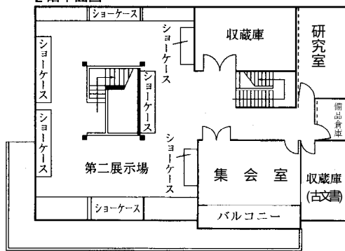
2階平面図
