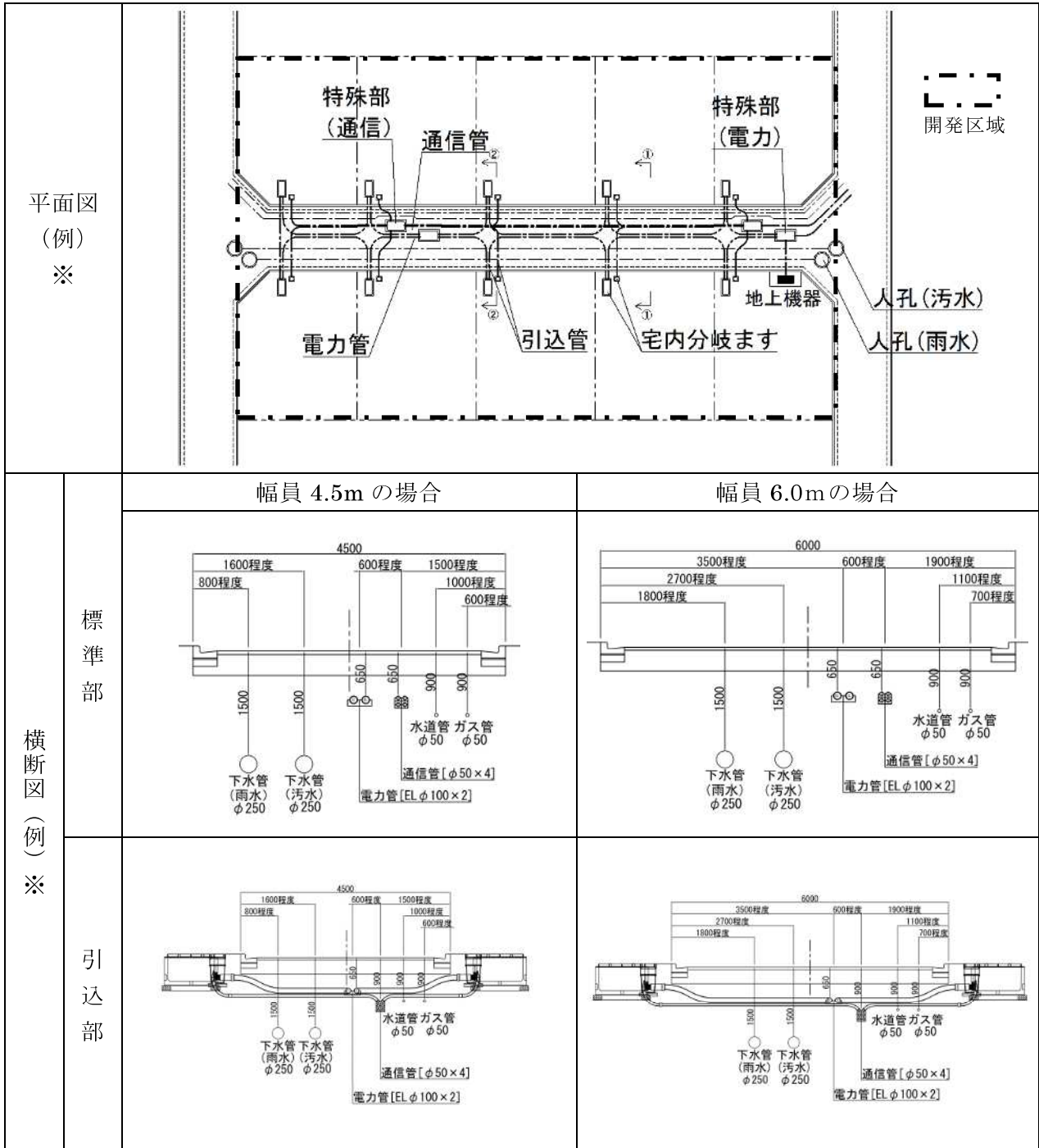
単独地中化方式 参考図
