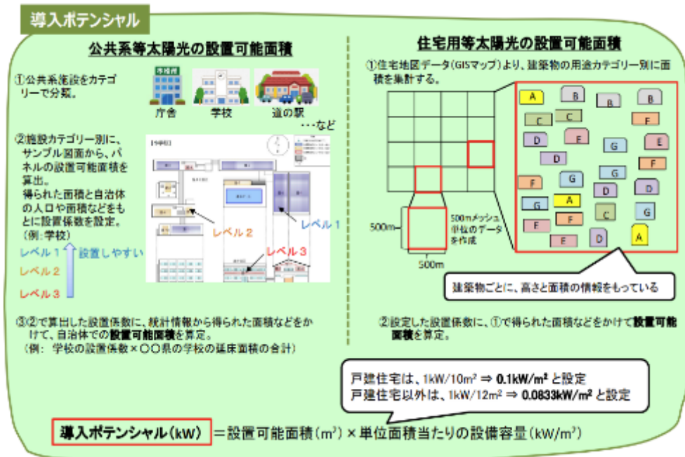
図7 REPOS における太陽光導入ポテンシャルの算定方法
