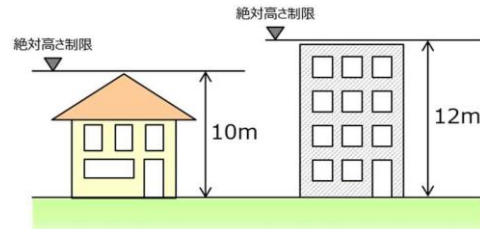
図 5 第一種低層住居専用地域等内における高さ（絶対高さ）制限のイメージ
