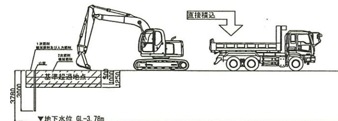
2-2`断面
