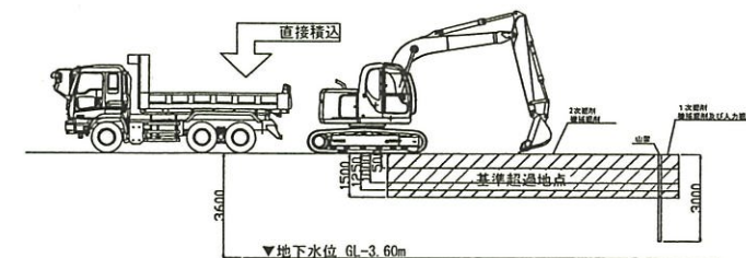
1-1`断面
