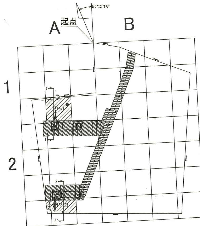
平面図 S=1:500
