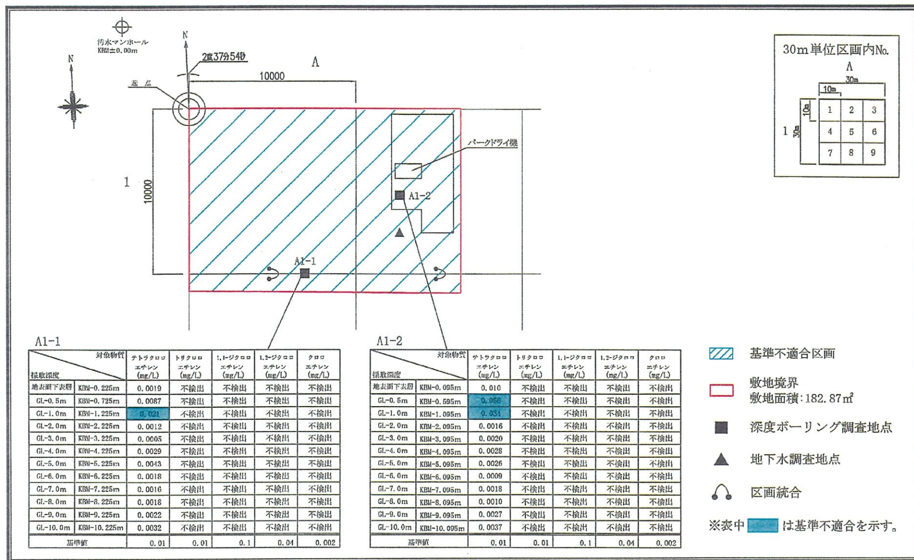
図-4 深度ボーリング調査結果図
