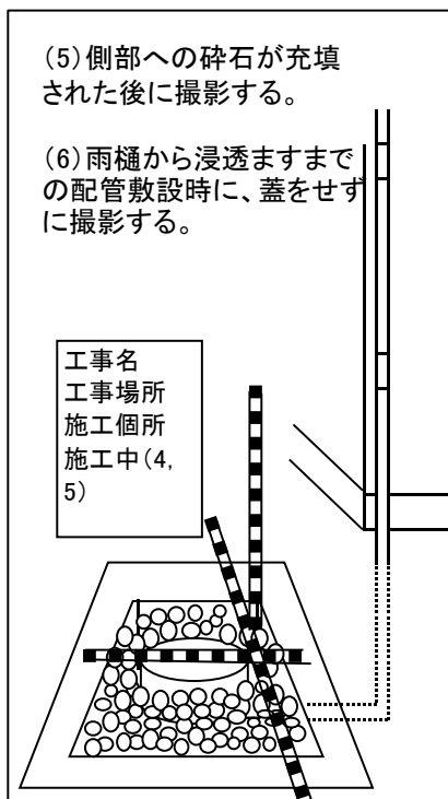
(5) (6) 施工中
