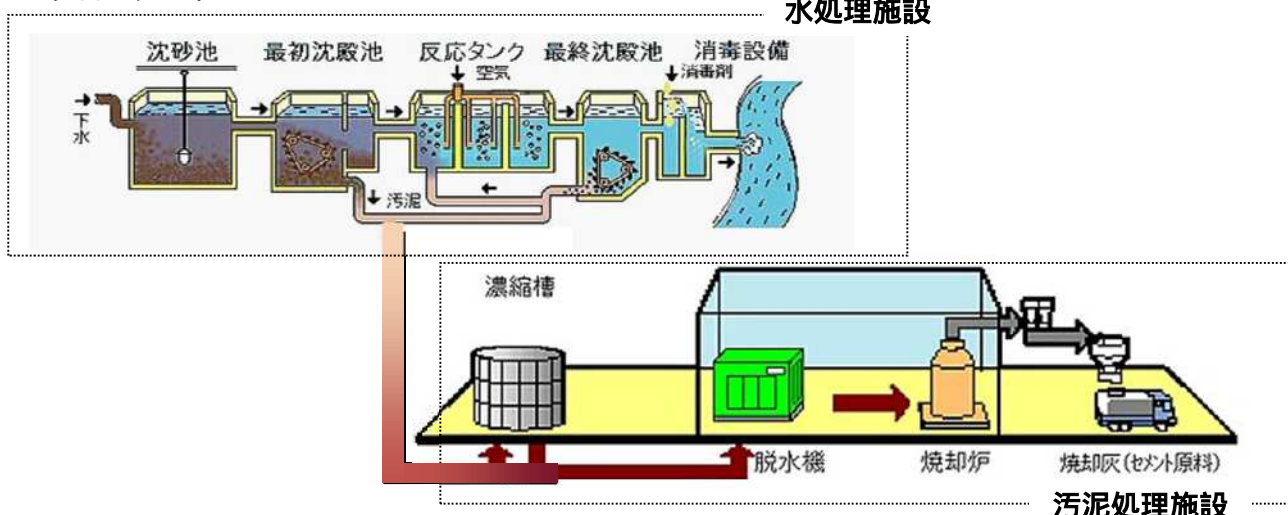
フローシート
