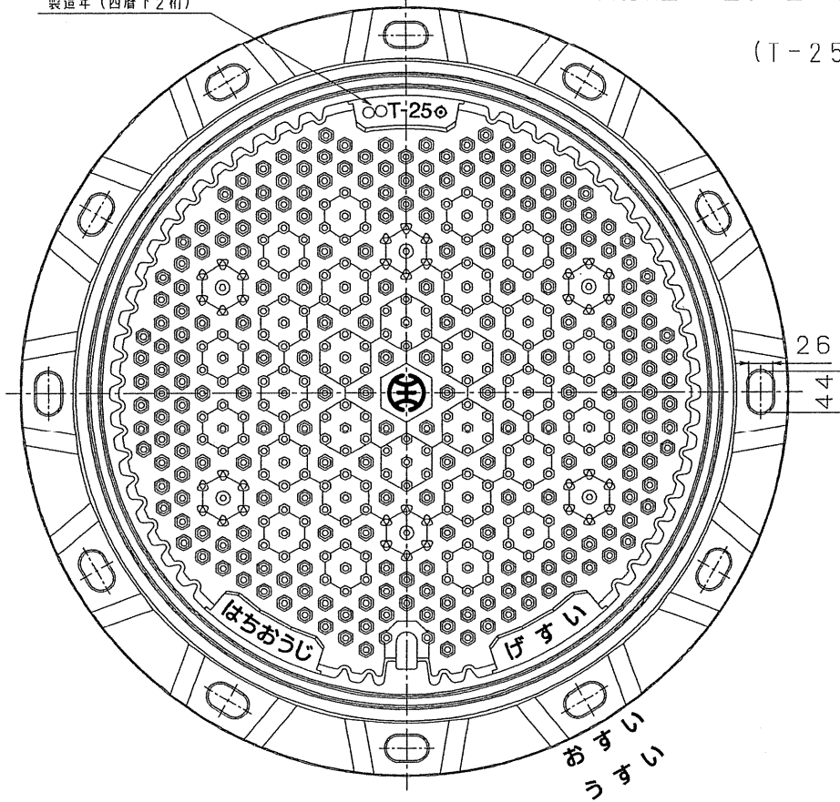
ふた, 枠平面図
