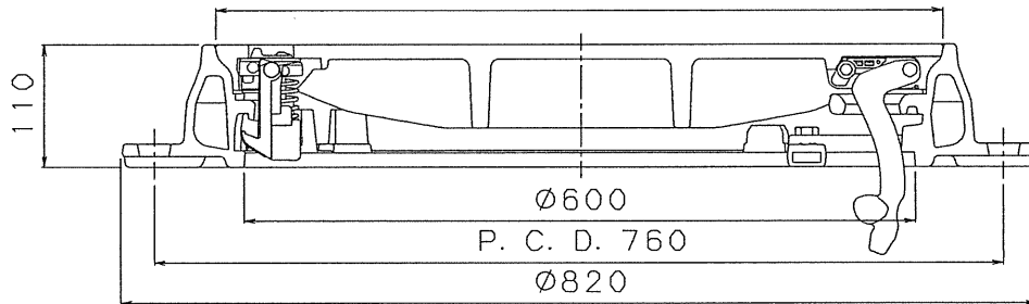
ふた, 枠断面図
