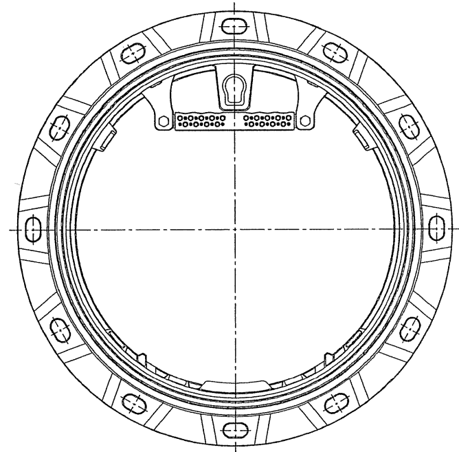
枠平面図
