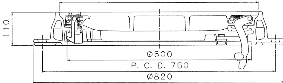
ふた，枠断面図
