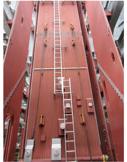
ボイラ据付状況
