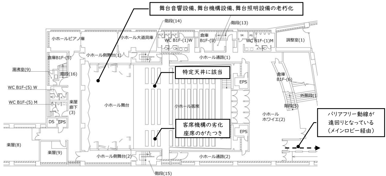
図 7-3 【現況】小ホール平面図
