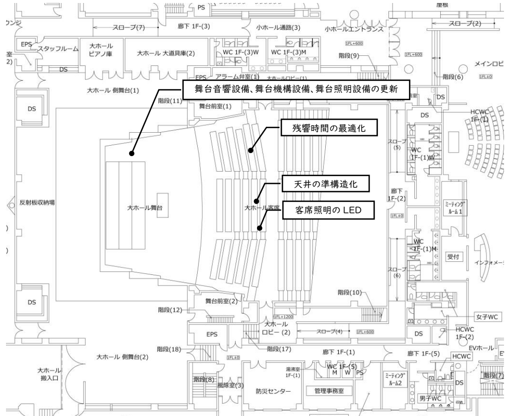
図 7-1 【改修案】大ホール概略図
