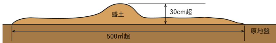
図 1-19 盛土又は切土する土地の面積が 500m 2 超で、盛土又は切土をする前後の地盤面の標高の差が 30cm 超となる場合イメージ
