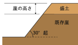
図 1-10 崖の高さ（盛土）
