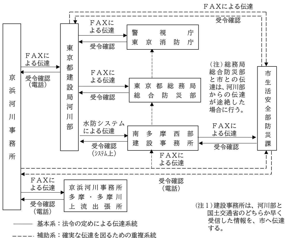
水防警報伝達系統図
