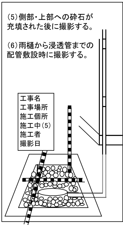
(5)(6) 施工中
