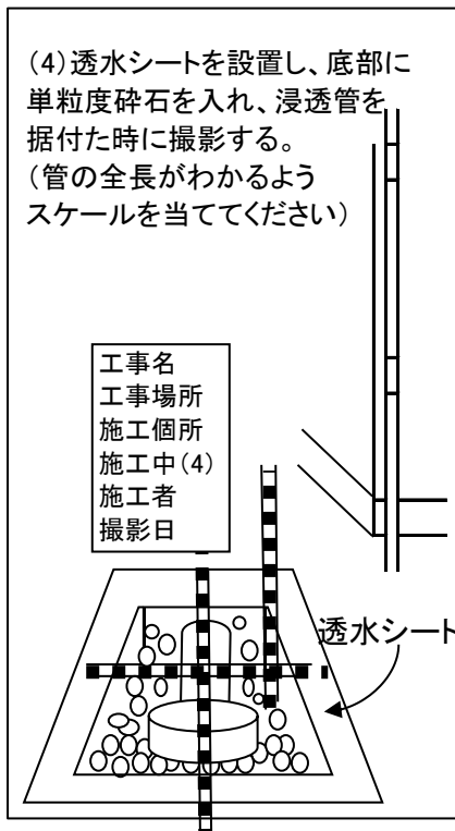
(4) 施工中
